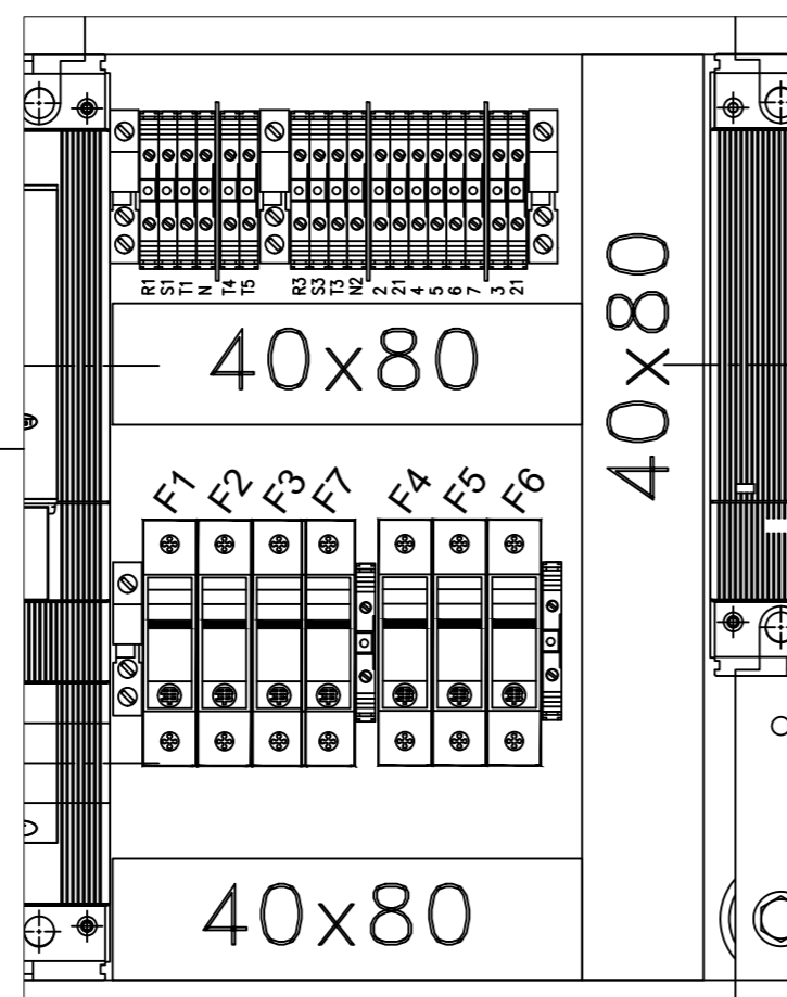
VISTA FRONTAL SIN PUERTA CON CONTRATAPA
