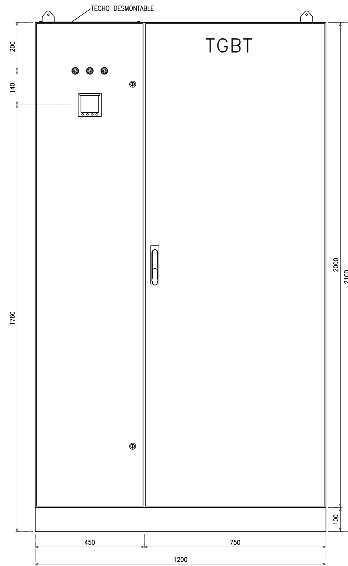
VISTA FRONTAL CON PUERTA
