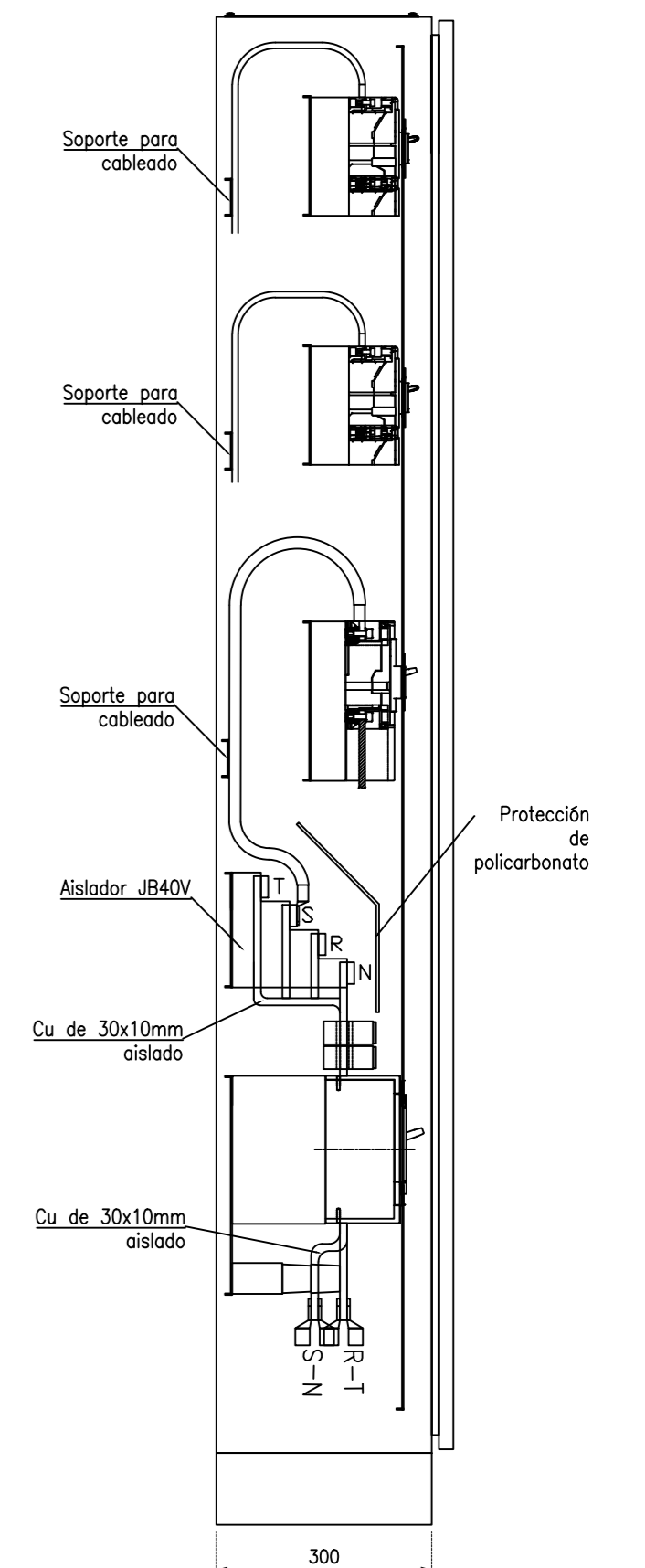
CORTE LATERAL
